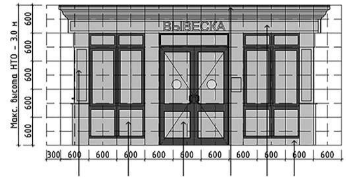
ДЕКОР ОСТЕКЛЕНИЕ ВХОДНАЯ ДВЕРЬ КАРНИЗ ФРИЗ ЦОКОЛЬ
