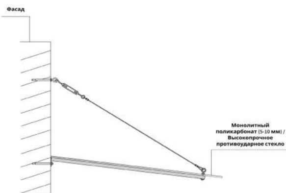
Вид сбоку
