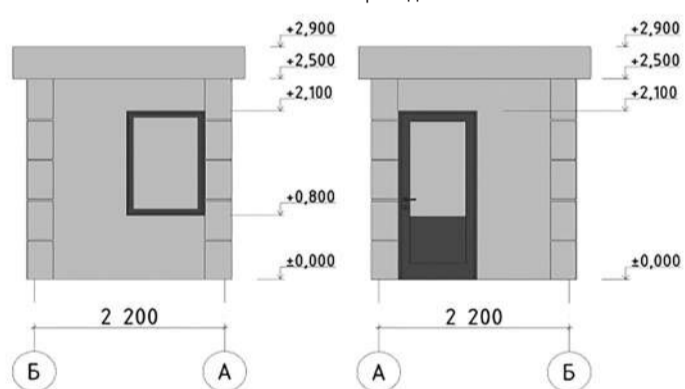
Проекция
