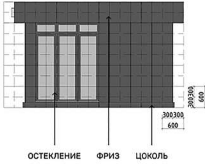
Боковые фасады
