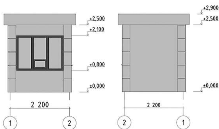
Боковые фасады
