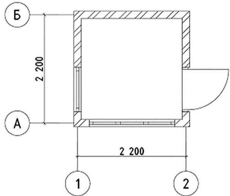
План Главный и задний фасады
