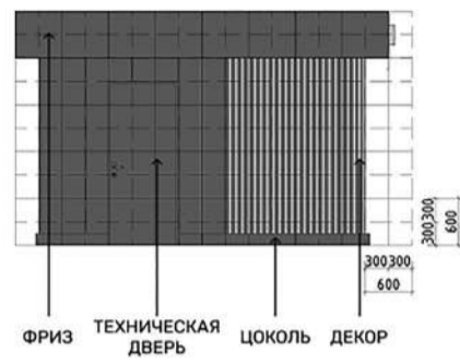
Проекция
