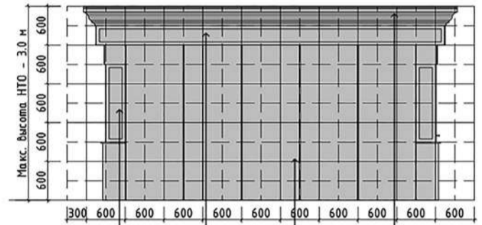
Задний фасад
