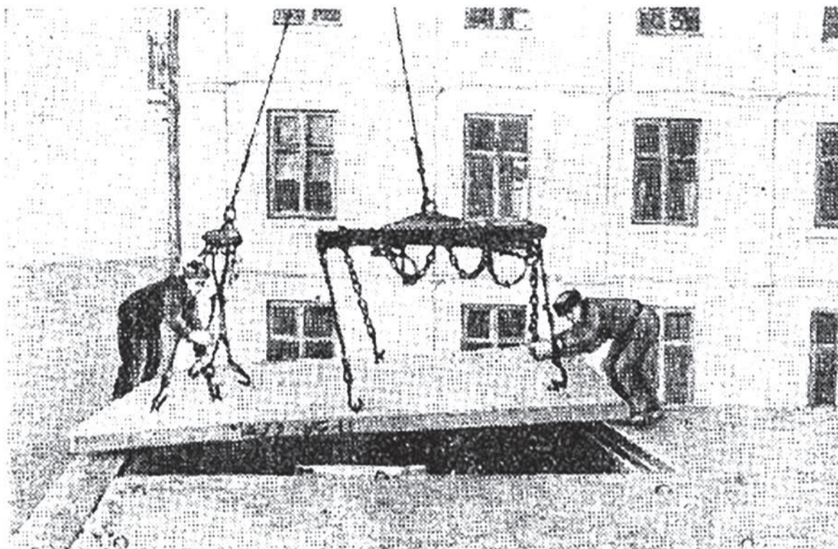
📷 / ФОТО: ОТКРЫТЫЕ ИСТОЧНИКИ, БРОШЮРА «КРУПНОПАНЕЛЬНЫЕ БЕСКАРКАСНЫЕ ДОМА (ОПЫТ СТРОИТЕЛЬСТВА В МАГНИТОГОРСКЕ)» 1955 Г.
